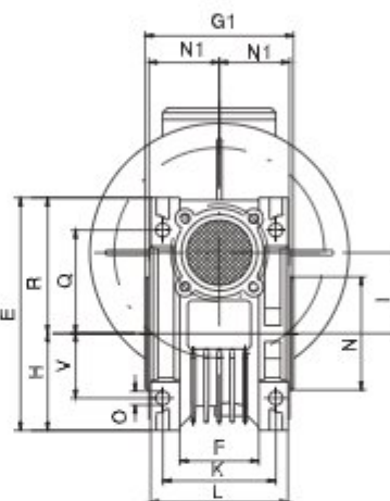
RV30-130
